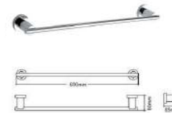
91201 Single rod 单杆 表面处理: 黑色 / 抛光 / 拉丝 材质: 304 不锈钢
